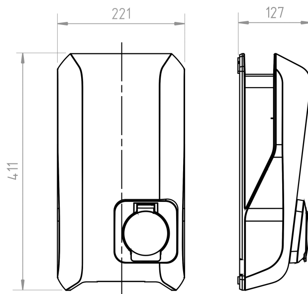
Abmessungen in Millimeter
